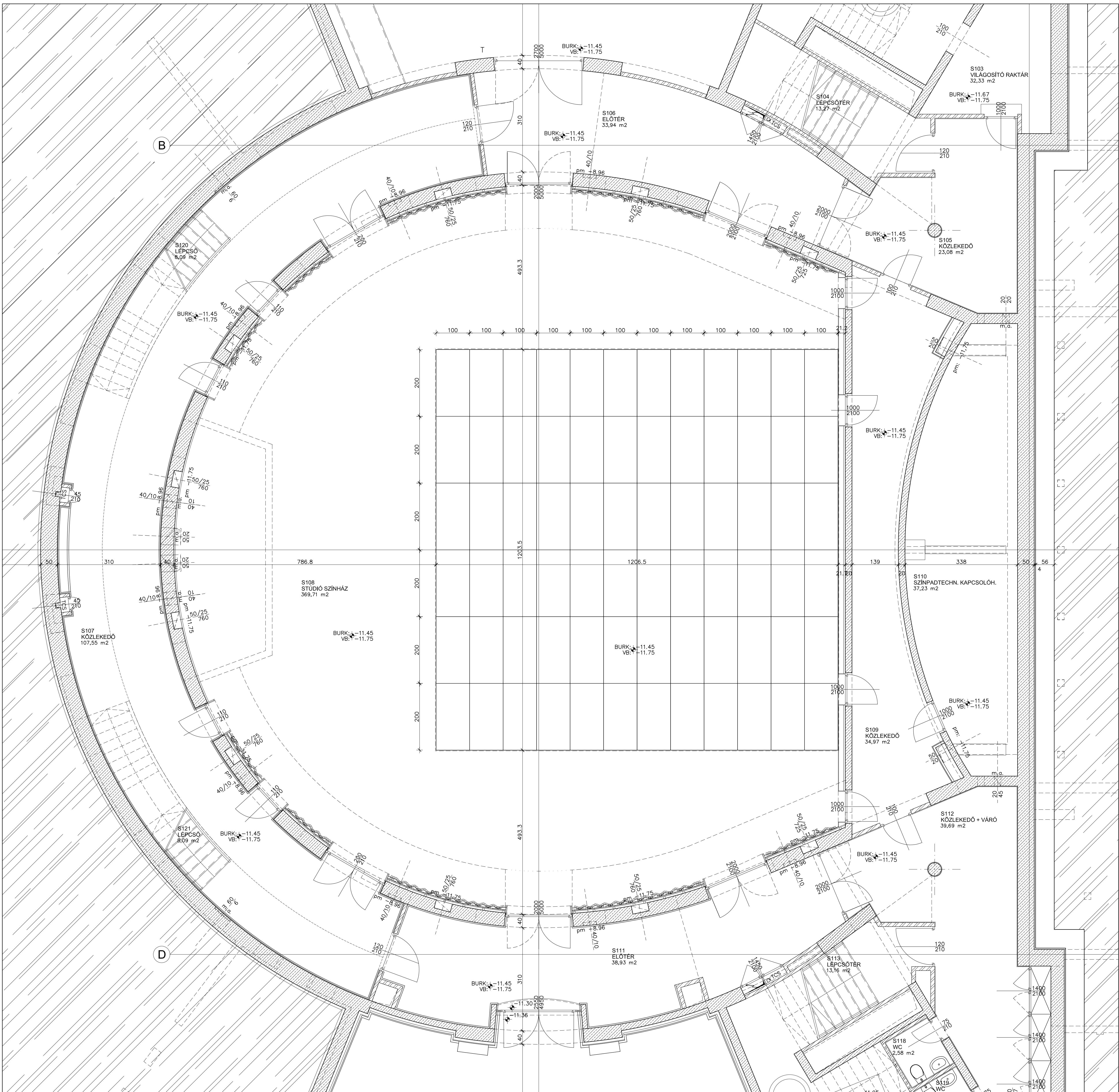
NEMZETI SZÍNHÁZ - STÚDIÓSZÍNPAD ALSÓGÉPÉSZET - P3 PINCE SZINTI ALAPRAJZ - M = 1 : 50 - 2001. NOVEMBER
