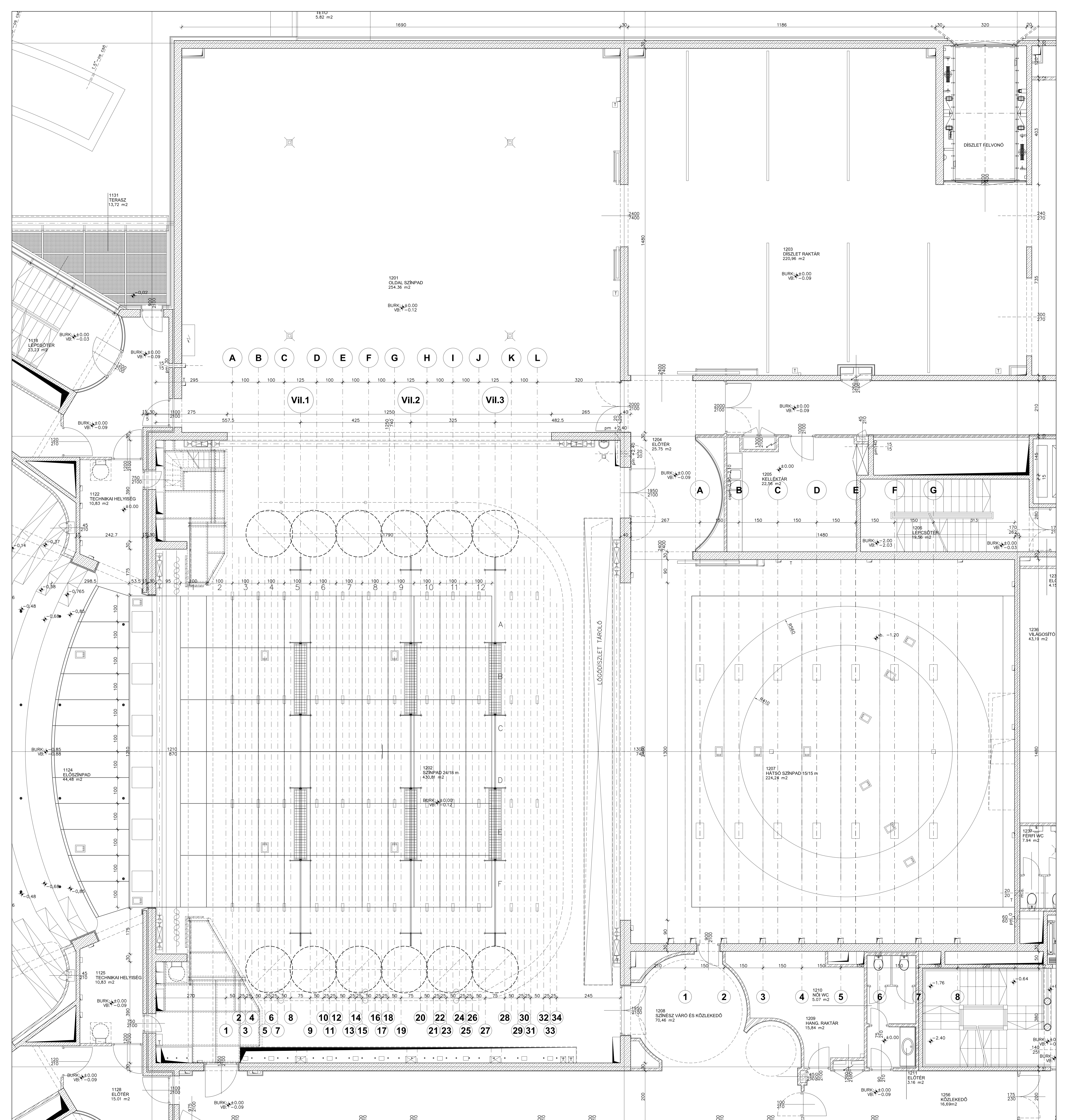
NEMZETI SZÍNHÁZ - SZÍNPAD, HÁTÓSÓ SZÍNPAD, OLDALSZÍNPAD I. EMELETI ALAPRAJZA - M = 1 : 50 - 2001. NOVEMBER
