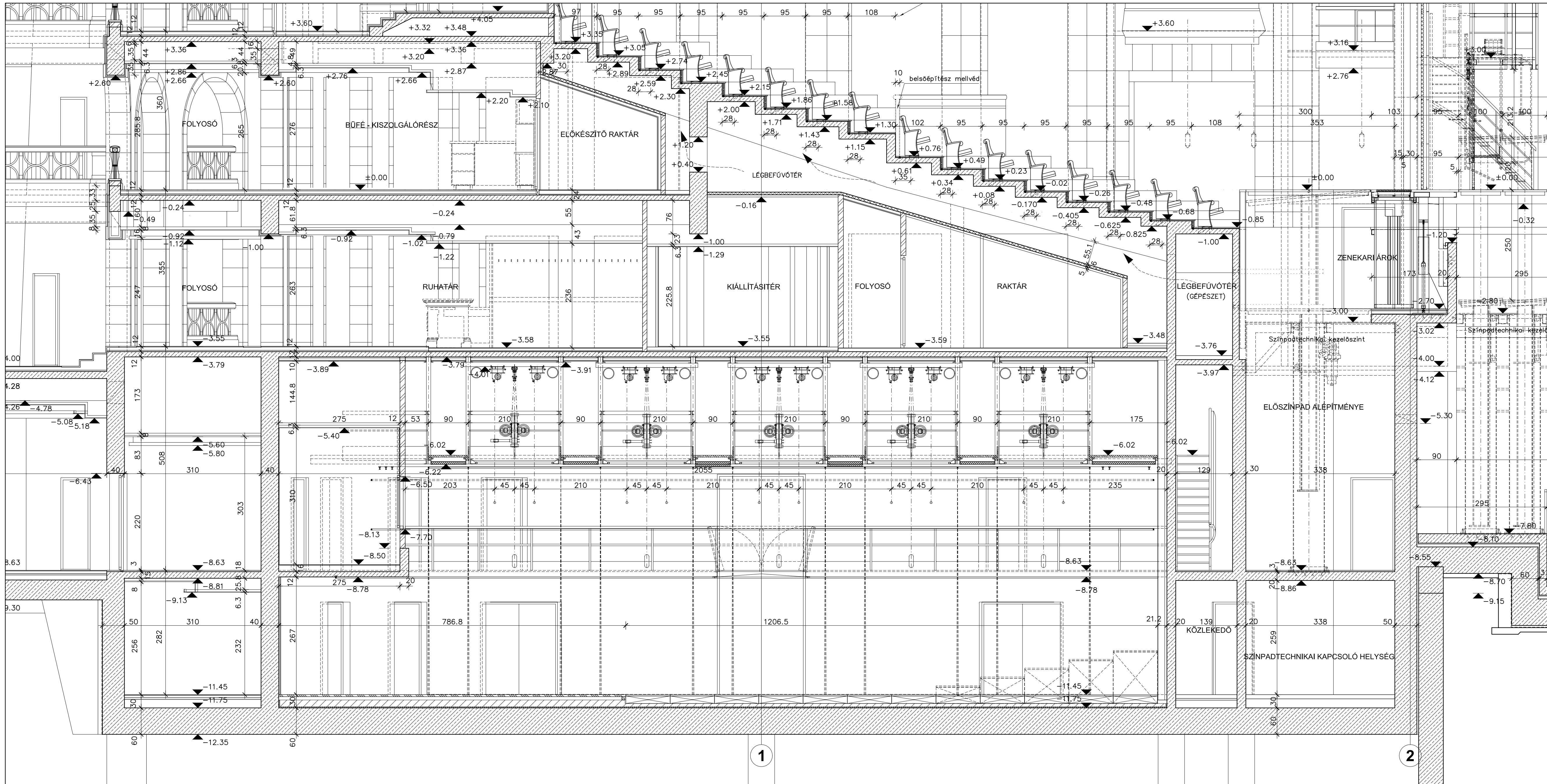
NEMZETI SZÍNHÁZ - STÚDIÓSZÍNPAD, ALSÓ-, FELSŐ-GÉPÉSZET - A-A HOSSZMETSZET - M = 1 : 50 - 2001. DECEMBER
