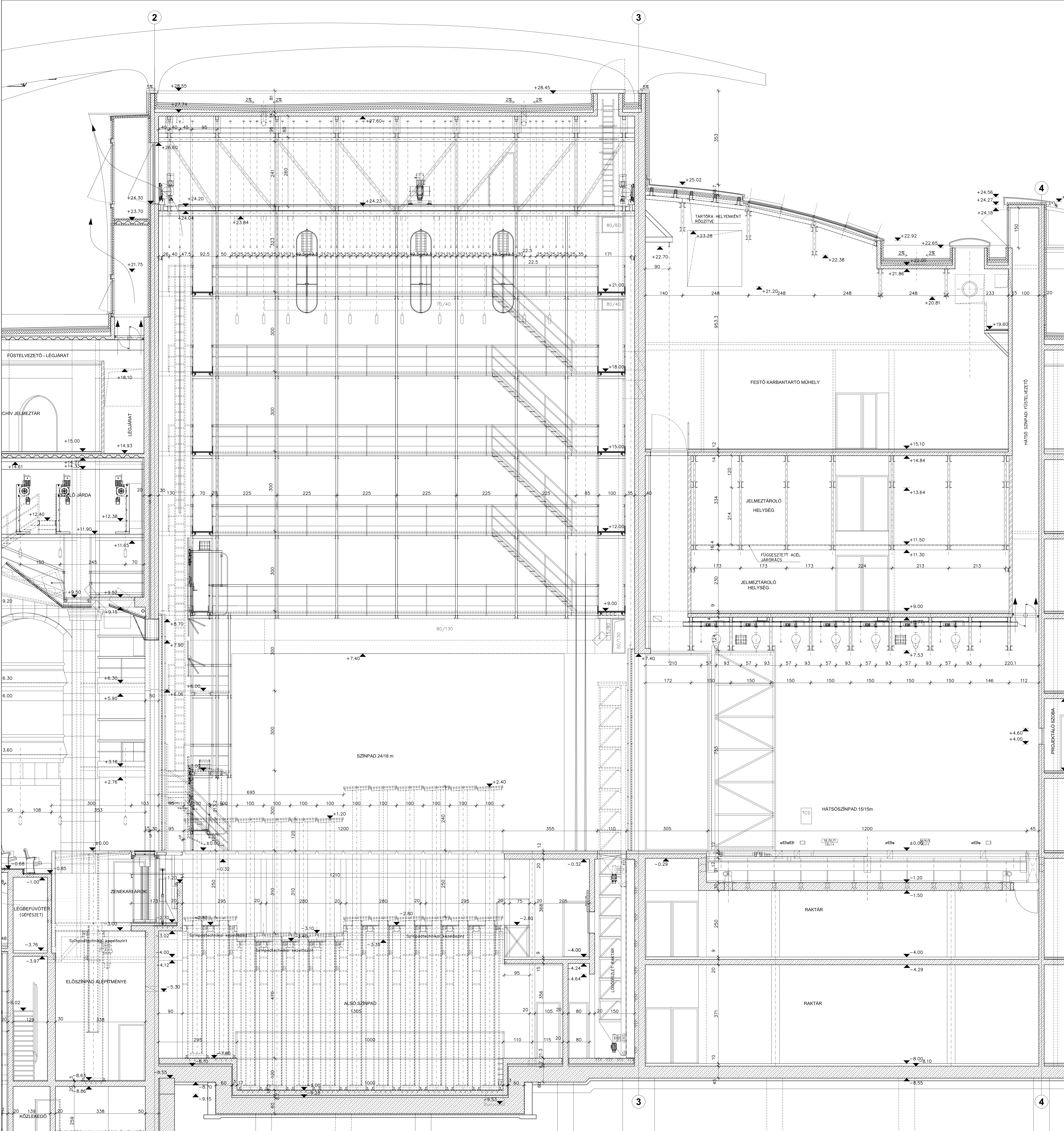
NEMZETI SZÍNHÁZ - SZÍNPAD, HÁTÓSZÍNPAD, ALSÓ-, FELSŐ-GÉPÉSZET - A-A HOSSZMETSZET - M = 1 : 50 - 2001. NOVEMBER
